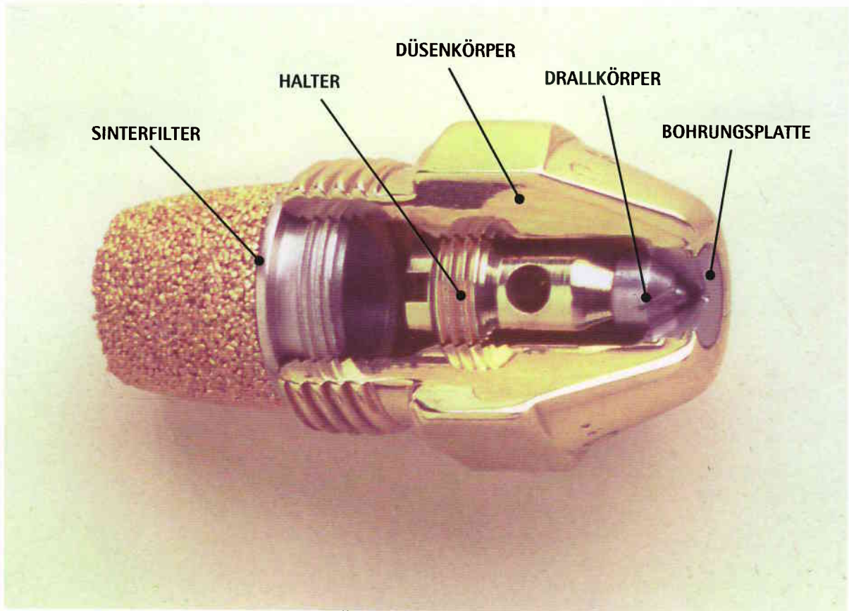
Öldüse ohne Düsenabschlußventil
