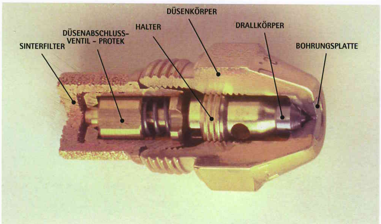
Öldüse mit Düsenabschlußventil
