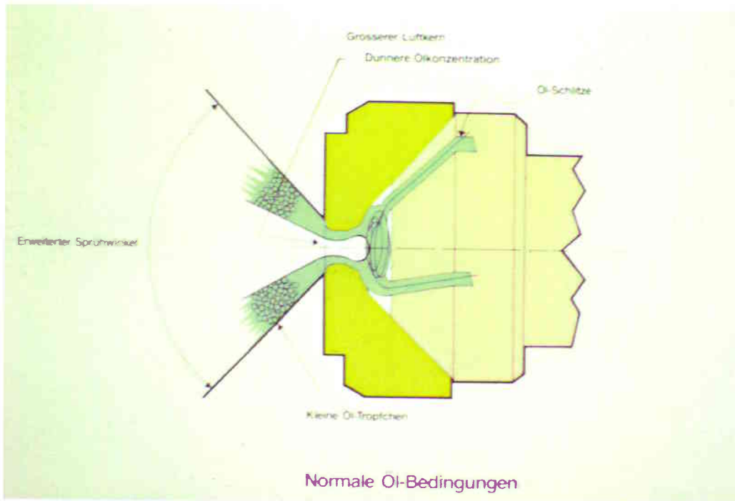
Schematische Darstellung der Vorgänge in der Drallkammer einer Öldüse
