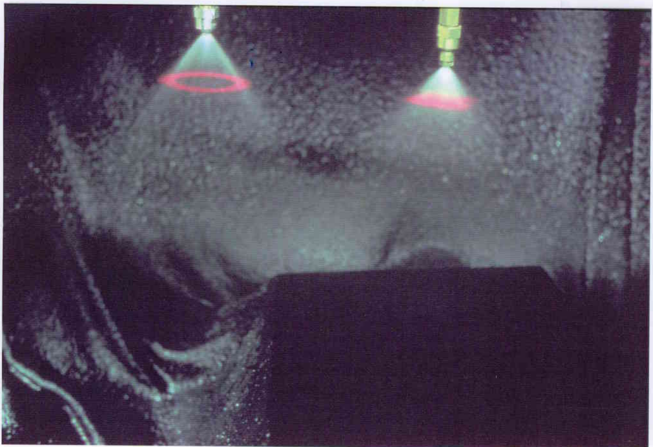
Reflexion des Laserstrahls (rot) bei einer Öldüse mit Sprühcharakteristik 'HOHL' (links im Bild) und 'VOLL' (rechts im Bild)
