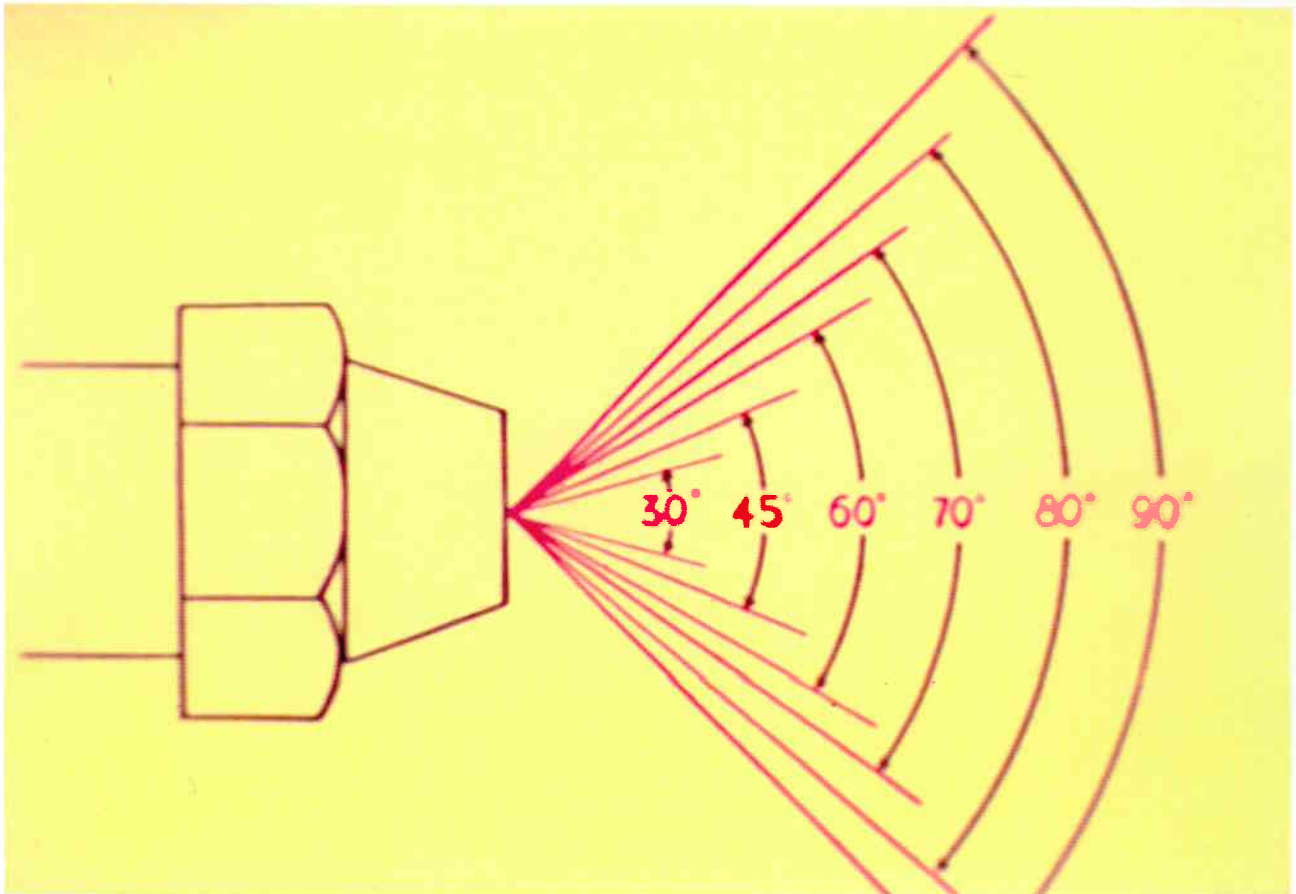
Darstellung der möglichen Sprühwinkel von Öldüsen
