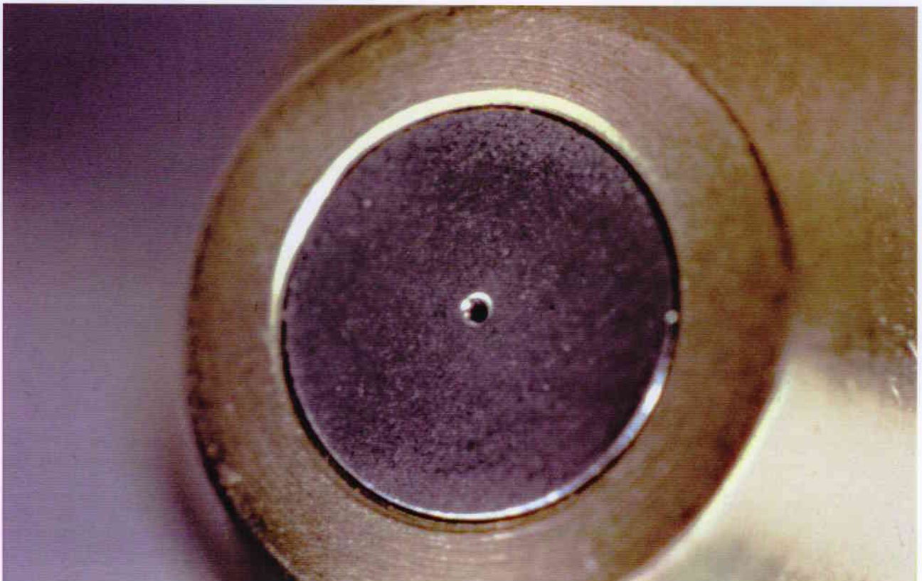
Draufsicht eines Düsenlochs. Erkennbar der Radius zur Erzeugung des Sprühwinkels (Lochdurchmesser: 200 \mu\text{m} )
